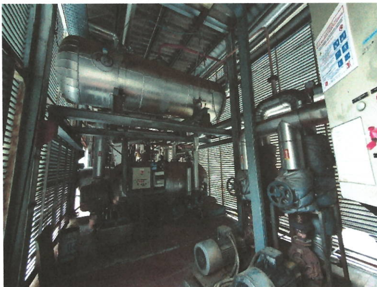
Foto 28: interno centrale termica – serbatoi olio
