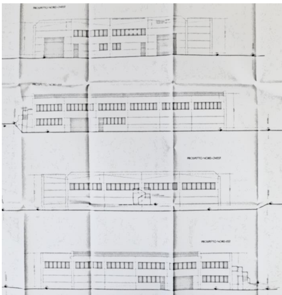
Prospetto da titolo edilizio
