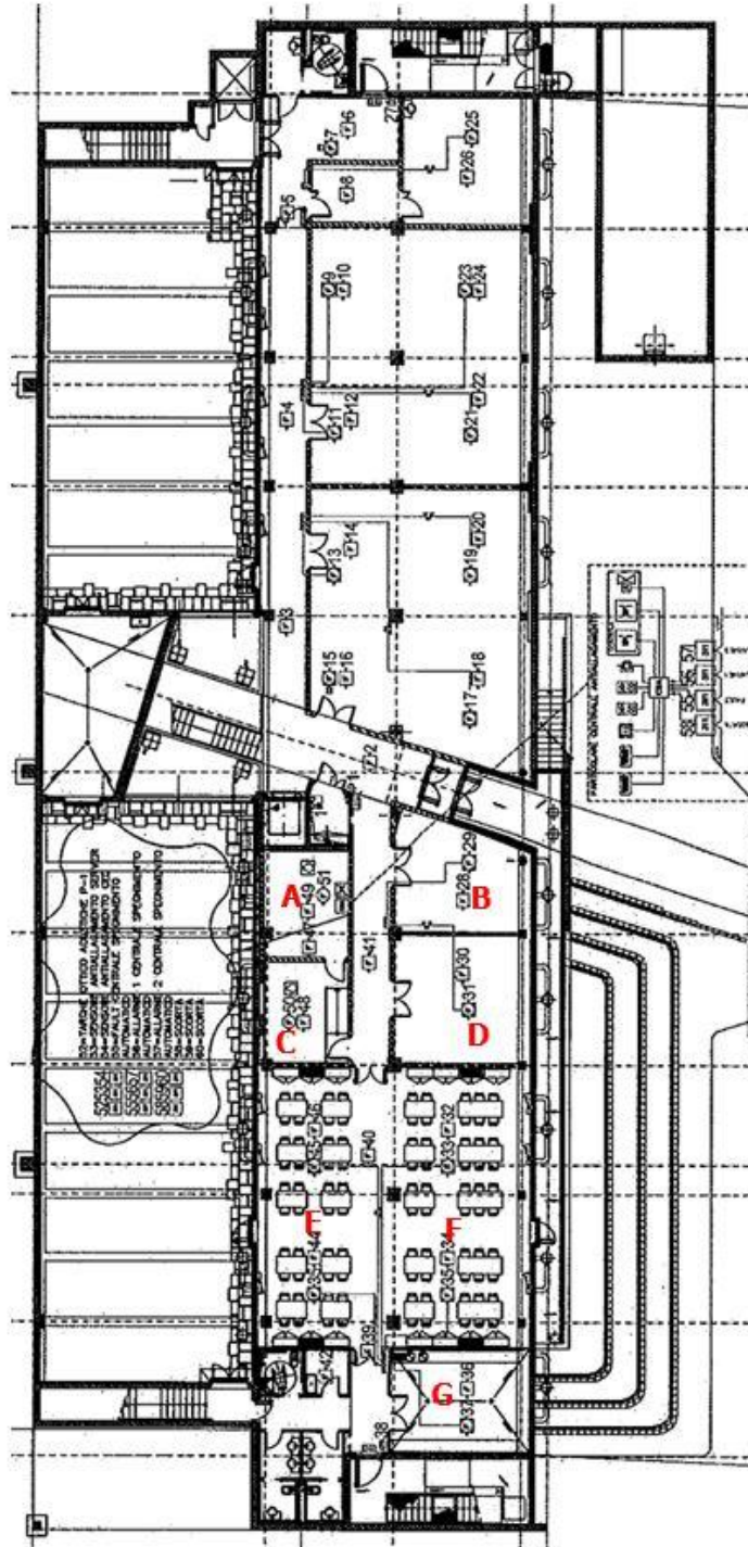
Figura 1: Piano seminterrato dell'ala uffici dello stabilimento della TMC ITALIA S.p.a. A) Locale server; B) Locale tecnico; C) Anticamera locale server; D) Ripostiglio attrezzature elettroniche; E) Sala mensa F) Sala meeting; G) Cucina.
