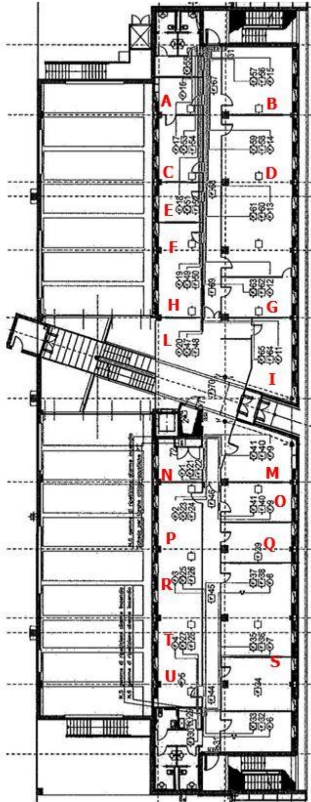
Figura 2: Piano rialzato dell'ala uffici dello stabilimento della TMC ITALIA S.p.a. A), D), E), F), G), H), M), N), O), P), Q), R), S), T) ed U) Uffici amministrativi; B) e C) Sale riunioni; L) Reception e sala d'attesa; I) Area accoglienza clienti; S) Ufficio tecnico.
